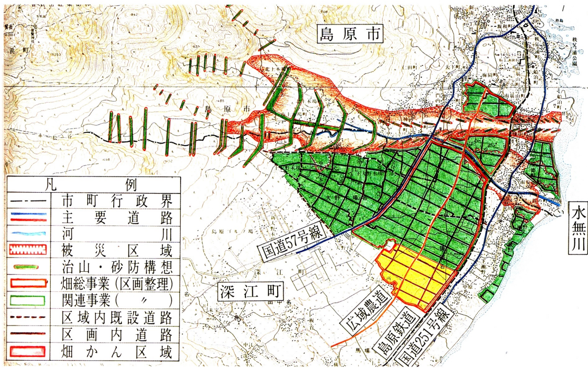
復旧・復興の事業計画平面図（長崎県農林部）
